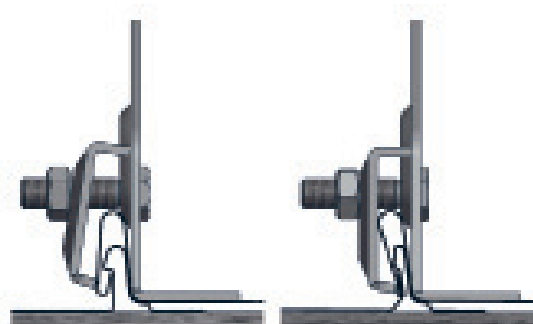
Lukkosaumakatto
